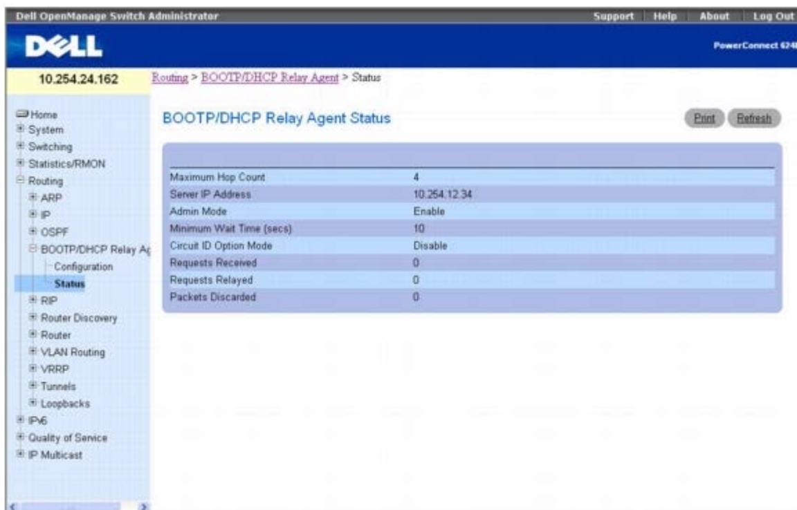
图 10-22. BOOTP/DHCP 中继代理状态
